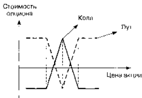
Рис. 8.3. Спред «бабочка»
