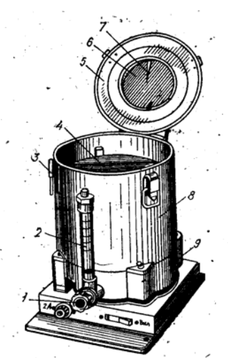
37- расм. Кротов апаратининг тузилиши:
