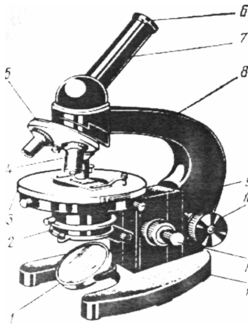
17-расм. Биологик микроскоп
