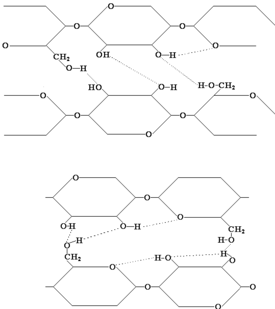
1.1-rasm. Mann va Marinar gipotezasi bo‘yicha sellyulozada hosil bo‘ladigan vodorod bog‘larni sxema.
