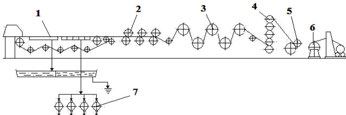
7.2-rasm. Tekis to'rli qog'oz quyish mashinasini texnologik sxemasi:
