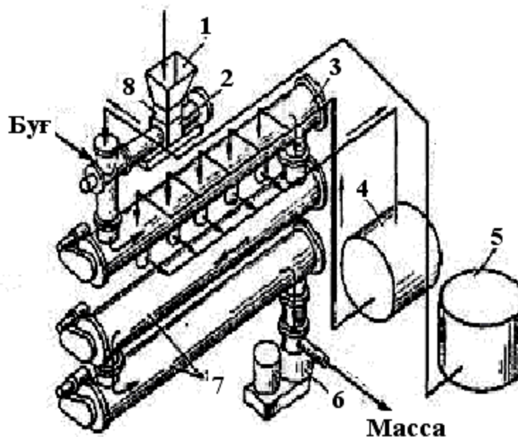
4.4-rasm. “Pandya” uzluksiz pishirish qozonli qurilma:
