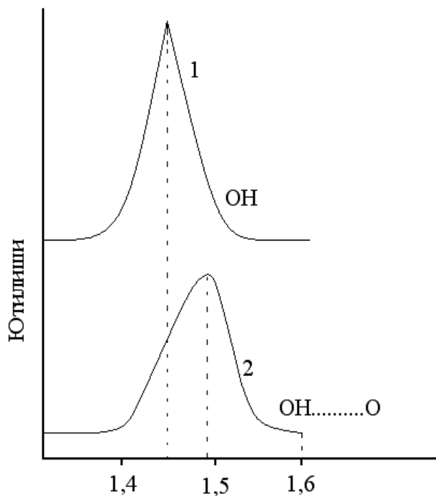
1.2-rasm. Ikkilamchi nitratni (1) va efirdan qayta olingan sellyulozani (regenerallangan) (2) spektrogrammasi.
