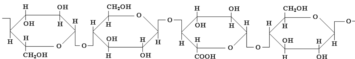
1.3-rasm. Aralashgan polisaxaridlarning tuzilishi.
