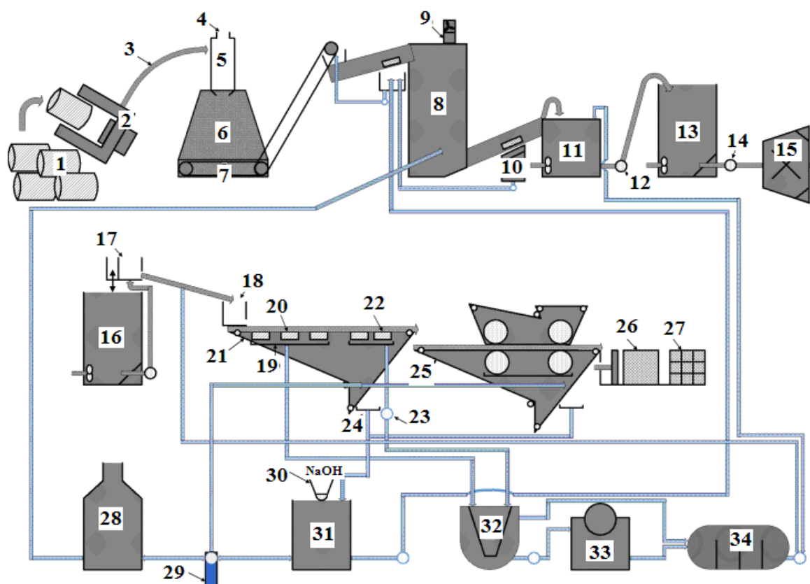
7.10-rasm. Uzlüksiz usulda somondan yarim tayyor sellyuloza olish texnologik sxemasi:
