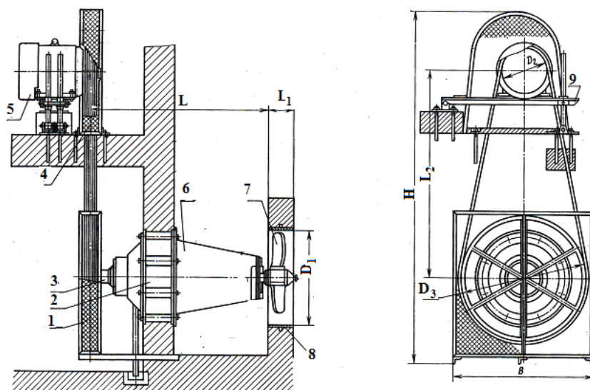
7.3-rasm. SU-750-13 markali sirkulyasiyalovchi qurilma:
