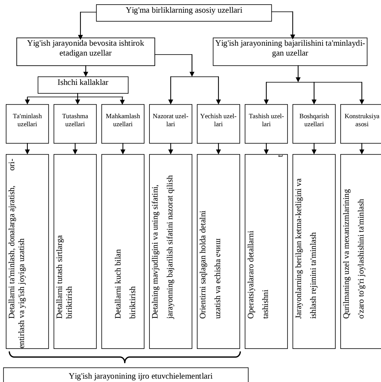
17.1-rasm. Avtomatlashtirilgan yig'ish uchun jihozlarni yaratishda hal qilinadigan masalalar sxemasining strukturasi
