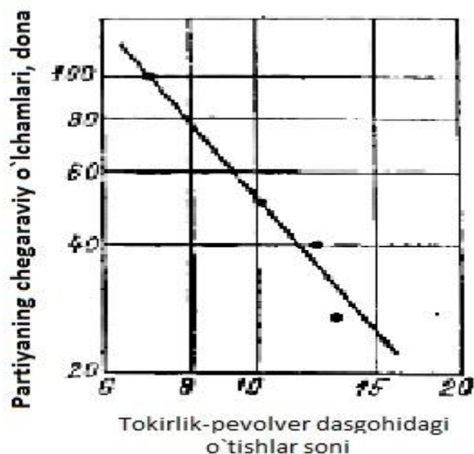
8.4-rasm. Zagotovkalarga ishlov berishni tokarlik-revolver dastgohidan bir shpindelli avtomatga o'tkazishni iqtisodiy samaradorligi chegaralari grafigi
