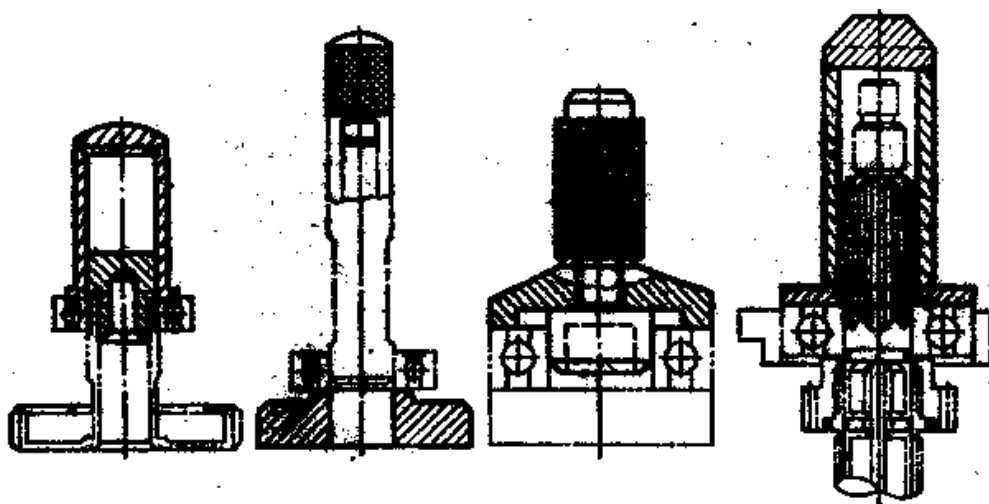
17.4-rasm. Zoldirli podshipnikni valga presslab o'rnatish uchun stakanlar va tutgichlar
