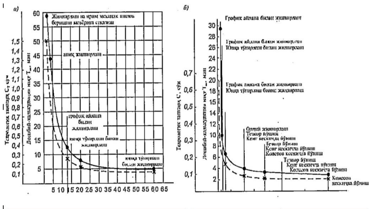
9.1-rasm Zagotovkalarga ishlov berish ish hajmi va tannarxining sirt aniqligi va g‘adir-budirligiga bog‘liqligi:
