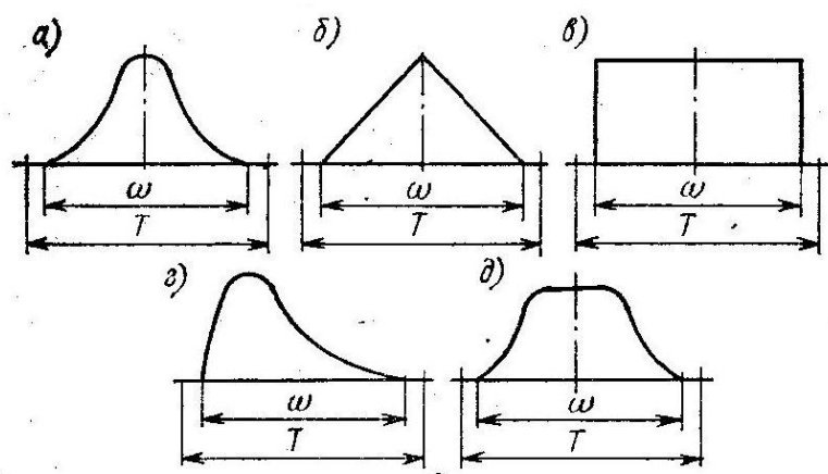
2.15-rasm. O'lchamlarning turli taqsimlanish qonunlari uchun zagotovkalarga nuqsonsiz ishlov berish sharti
