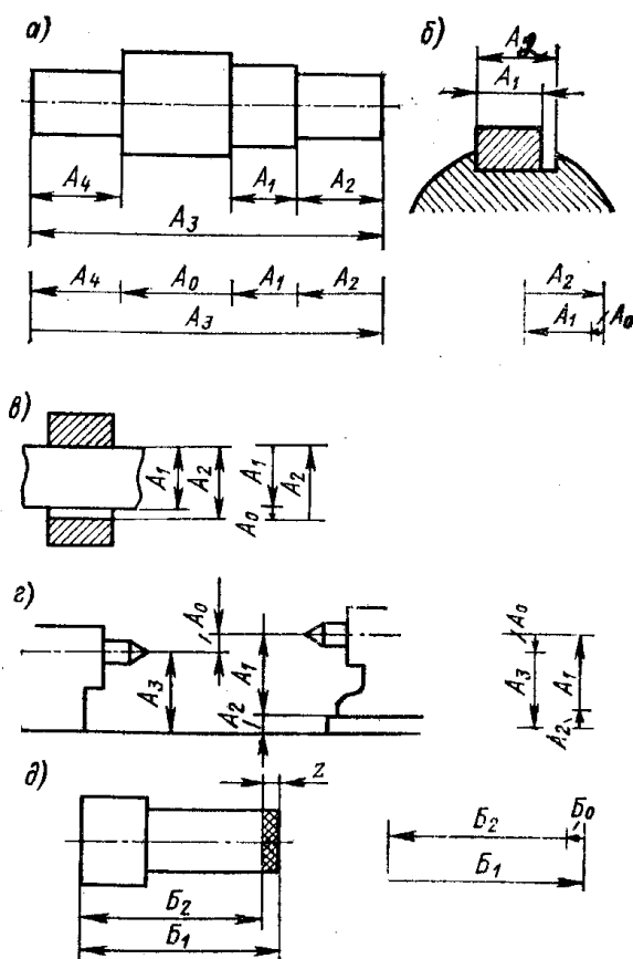
5.1-rasm. O'lcham zanjirlarining turlari
