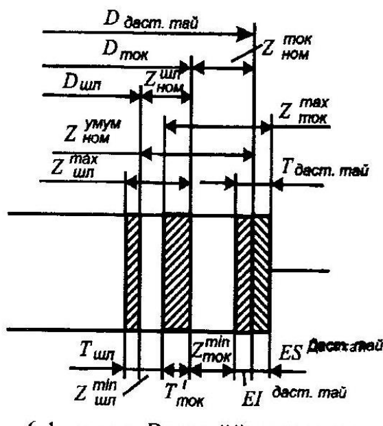
7.1-rasm. Valga yo'nish va jilvirlash orqali ishlov berishda qo'yimlarning va dopusklarning joylashish sxemasi
