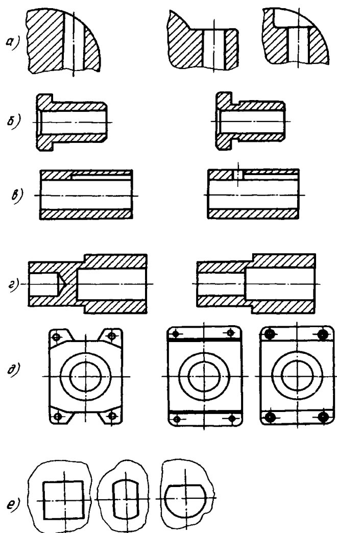
10.4-rasm. Notexnologiyabop va texnologiyabop konstruksiyali detallar namunalari
