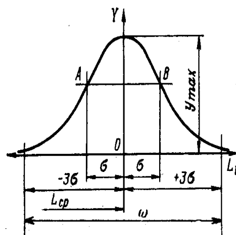
2.7-расм. О'лчamlar normal taqsimlanishining egri chizig'i (Гаусс қонуни)
