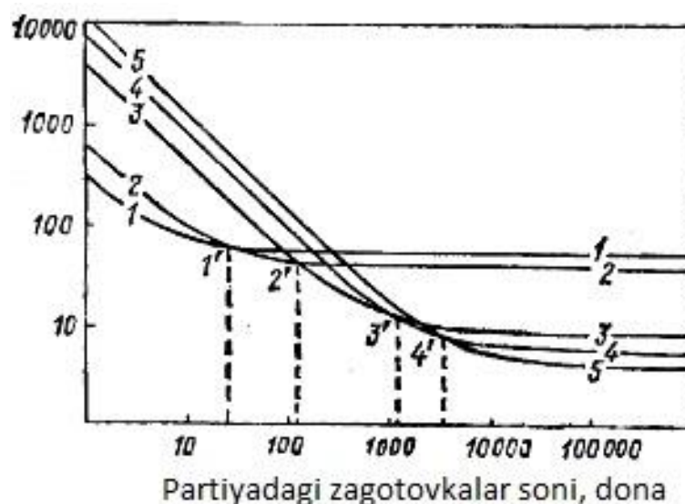
8.3 rasm. Pogʻonali vtulkalarni turli jihozlarda tayyorlashda tannarxning oʻzgarishi:
