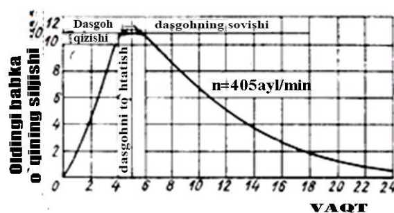
2.4 Rasim Toʻkriklik dastgohining markazida ishlov berishda oldingi babkaning qizishi natijasida uning oʻqining garizantal yoʻnalishi boʻyicha siljishi oldingi babka
