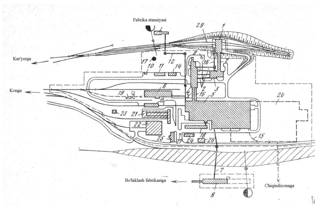
20-rasm. Katta ishlab chiqarish unumdorligiga ega flotatsiya fabrikasining bosh rejasi
