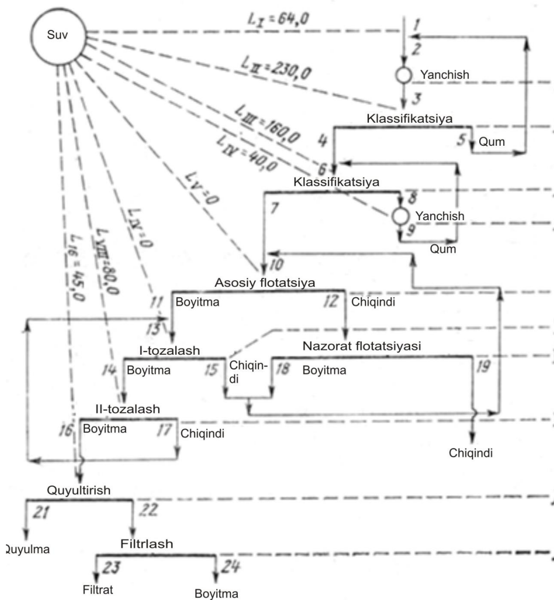
19-rasm. Suv sarfi sxemasini hisoblashga doir (15 va 18-mahsulotlarning yig'indisi 20-mahsulot, 1-tozalashga qo'shladigan suvning miqdori- L_{VI} )
