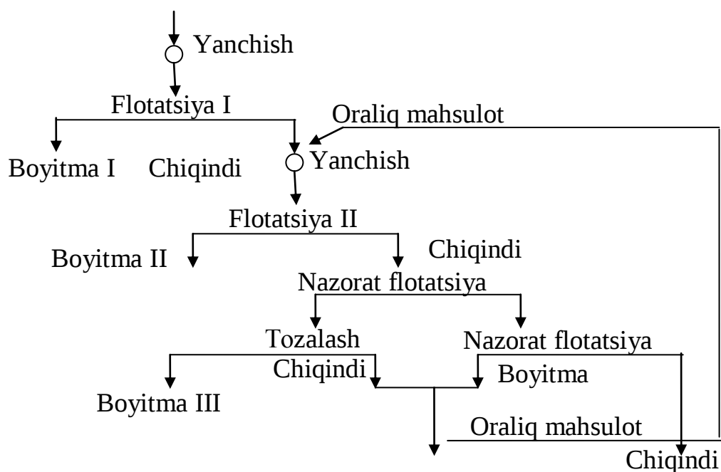
15-rasm Nazorat flotatsiyasi sonlarining ortishi yoʻnalishida rivojlanuvchi flotatsiya sxemasiga misol
