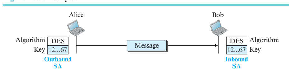
Figure 10.53 Simple SA
