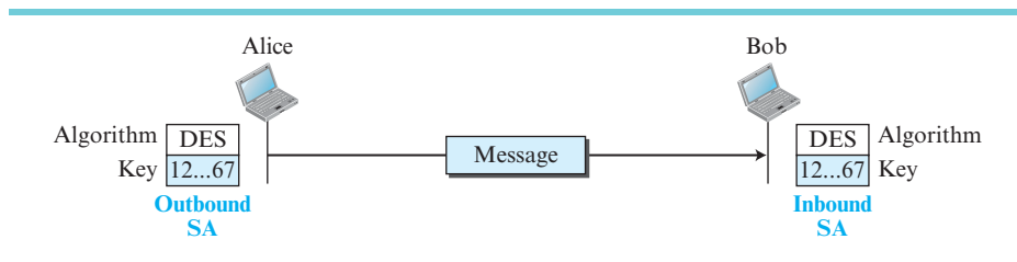
Figure 10.53 Simple SA
