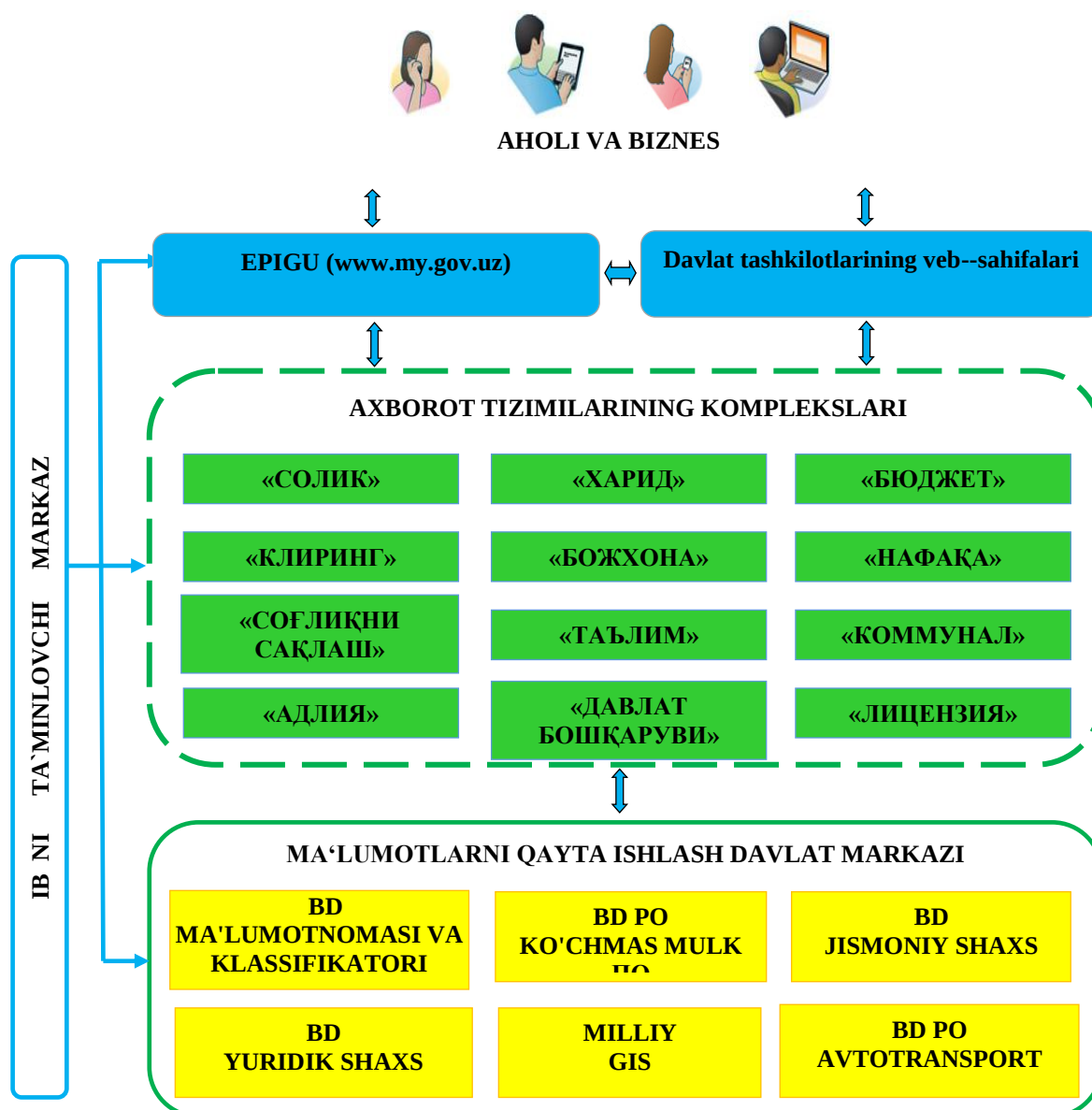
10.2-rasm. "Elektron hukumat" tizimining arxitekturas 105
