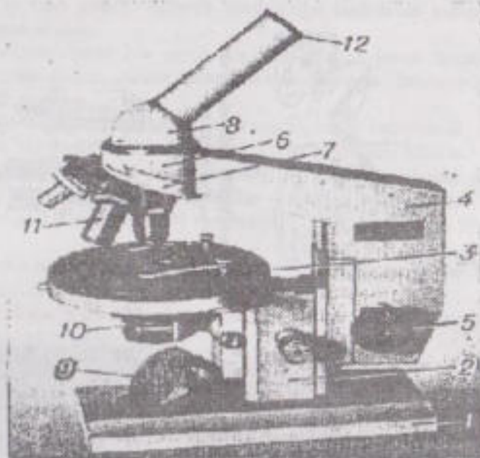
7-rasm. «Biolam» biologik mikroskopining tuzilishi: 1-asosi; 2-mikrovinti; 3-buyum stolchasi; 4-tubus tutqich; 5-makrovinti; 6-boshchasi; 7-revolver; 8-ko'rish o'rnatmasi uchun moslama; 9-ko'zgu; 10-kondensor; 11-obyektiv; 12-okulyar.
