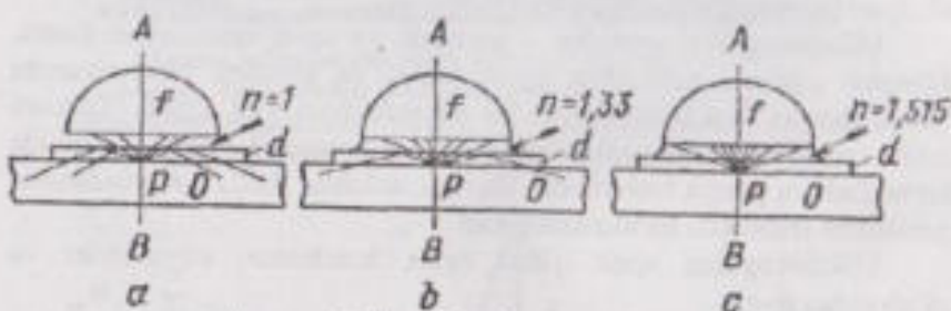
9-rasm. Optik mikroskopning obyektivlari:
