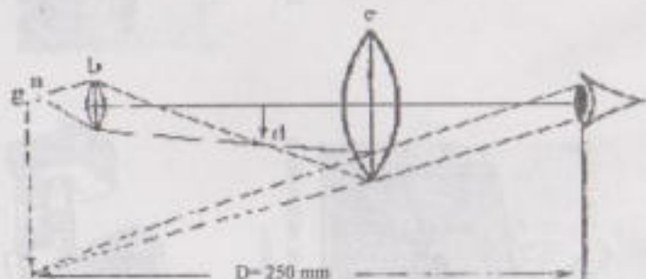
8-rasm. Mikroskopning optik sxemasi: a-obyekt; b-obyektiv linzasi; d-obyektning teskari ko'rinishi; e-okulyarning yuqoridagi linzasi; g-obyektning ko'rinadigan tasviri.
