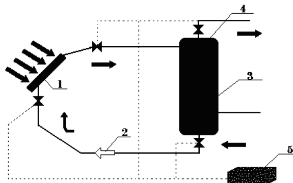
1a-rasm. Bir konturli qurilma tizimi sxemasi.
