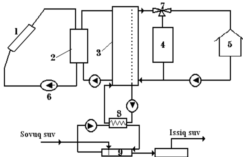
15- rasm. Isitish va issiq suv ta'minoti suyuqlik quyosh tizimining sxemasi.
