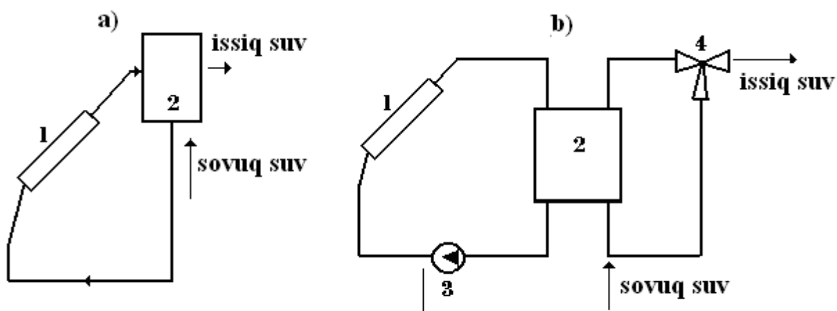
8-rasm. Quyosh suv isitish qurilmalarida tashuvchining (a) va majburiy (b) tsirkulyatsiyasining printsipl sxemasi
