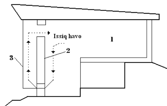
13-rasm. Passiv quyosh sistemasi bilan isitiladigan binoning oynalangan janubiy tomoni va issiqlik to'plagichi devori oralig'ida havoning tabiiy tsirkulyatsiyasi.
