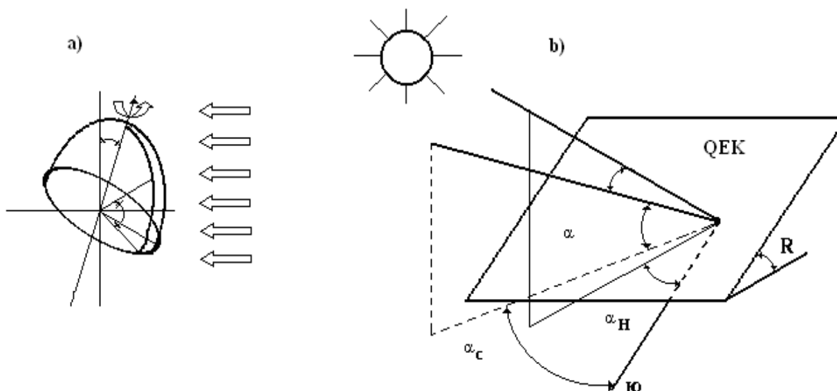
21-rasm. Er sathi va quyosh kollektorining yuzasini quyosh nurlariga nisbatan joylashishini xarakterlovchi burchaklar.
