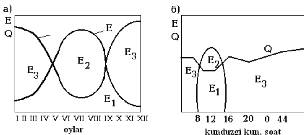
25-rasm. Yil (a) va sutka (b) davomida tushayotgan quyosh energiyasi E va binoni issiqlik bilan ta'minlash quvvati, Q miqdorlarining o'zgarishi
