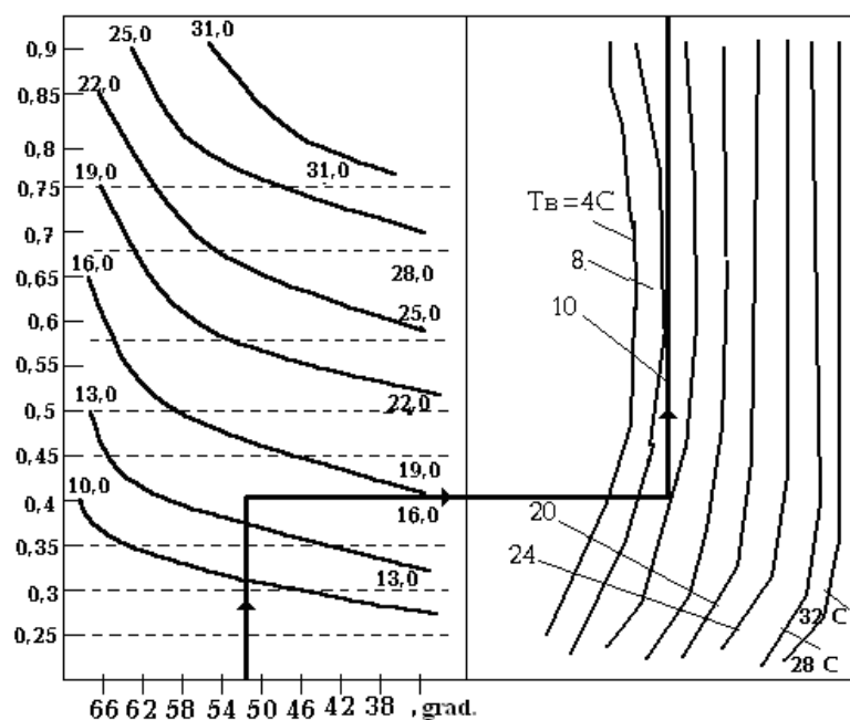
29-rasm. Mavsuniy quyosh issiqlik sistemalari uchun QEK yuza maydonini aniqlash monogrammasi.
