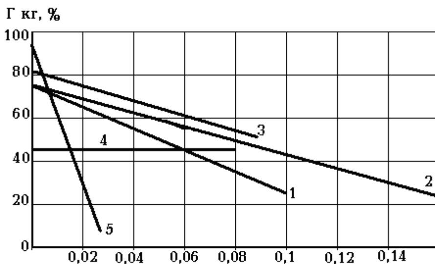
24-rasm. Quyosh energiyasi kollektorlari turlarining tavsifnomalari.
