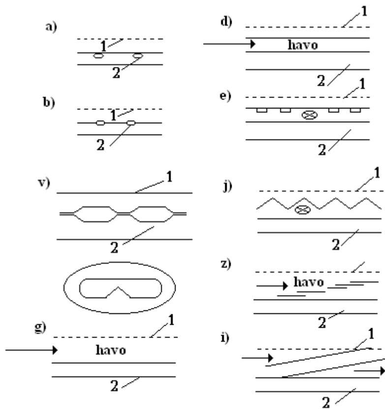
22 -rasm. Suvli va havoli quyosh energiyasi kollektorining tizimlari
