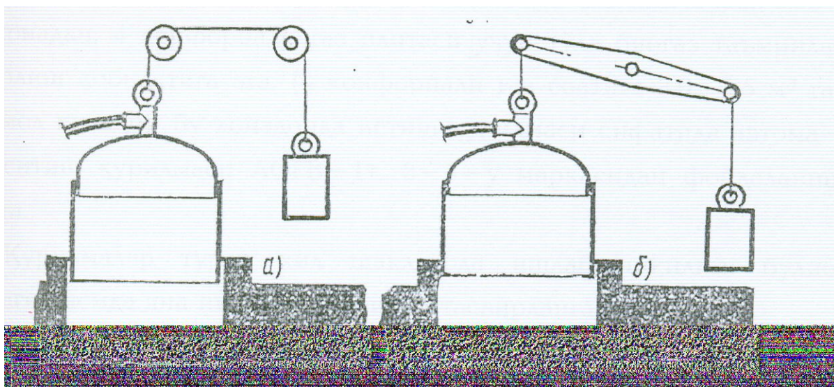
28-rasm. Muvozanatni saqlash qurilmasi
