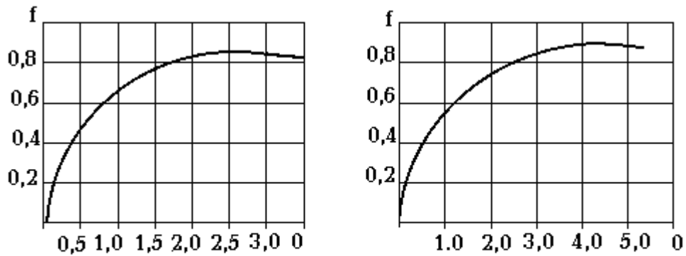
26-rasm. Quyoshli isitish tizimi uchun issiq suv ta'minoti (a) va isitish va issiq suv ta'minoti (b) f dan Q ga umumlashtirilgan bog'liqlik grafiqi.
