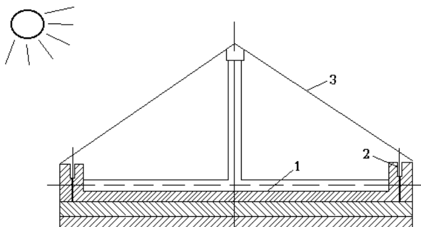
10-rasm. Parnik konstruksiali sho`rsizlantirish qurilmasi.
