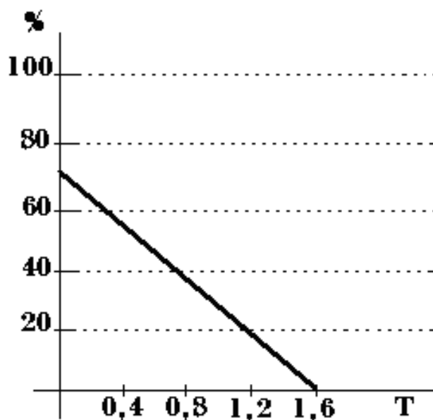
7-rasm. Quyosh kollektorining ishini navsiflovchi egri chiziq.
