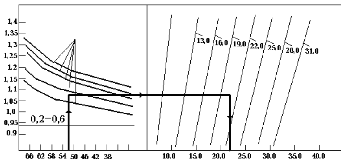
28 -rasm. Kollektor yuzasiga bir necha kunduzda tushayotgan energiyasining o`rtacha miqdorini hisoblash nomogrammasi.
