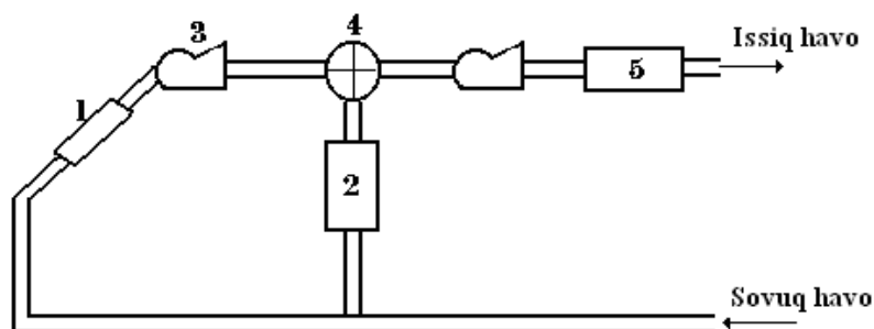
14-rasm. havoni isituvchi quyosh qurilmasi tizimining printsiptial sxemasi.
