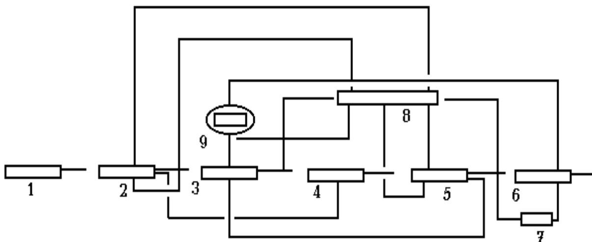
20-rasm. Quritish rejimini boshqaruv blokiga ega bo'lgan quyosh havo issiqlik generatori tizimi.
