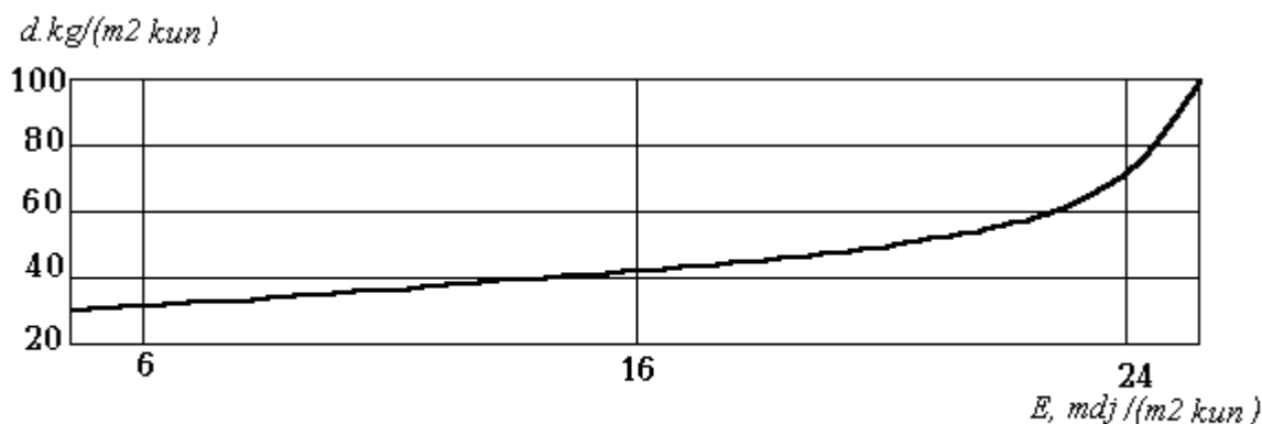
27- rasm. Gorizonttal yuzaga tushayotgan quyosh energiyasining sutkalik umumiy miqdori E bilan quyoshli issiq suv ta'minoti sistemasining sutkalik birlik unumdorligi d o'rtasidagi bog'liqlik.
