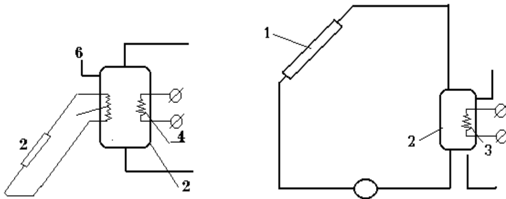
9-rasm. Ikki konturli quyosh suv isitish qurilmalarida issiqlik tashuvchining (a) va (b) majburiy tsirkulyatsiyasining printsipl sxemasi.
