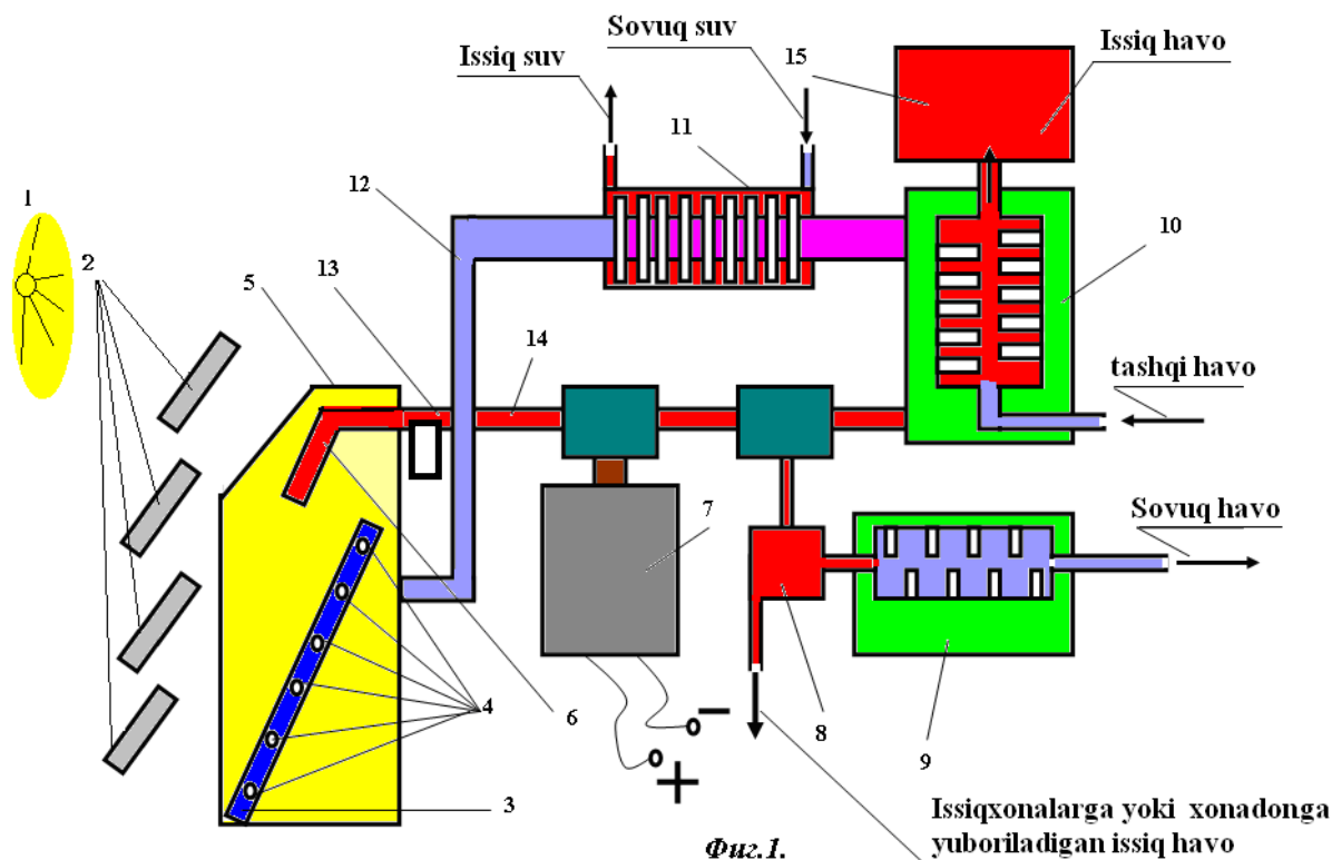
1-rasm. Ko`p funktsiyali quyosh qurilmasining printsiplial ishlash sxemasi.
