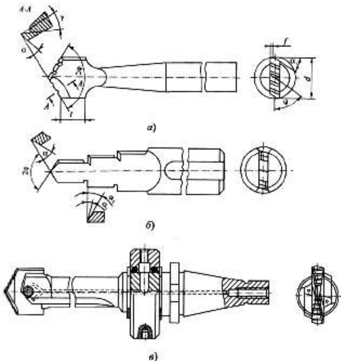
3.1-rasm. Peroi (kurakchasimon) parmalar:
