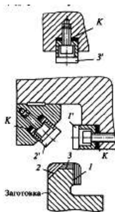
7.7-rasm. Tashqi sidirgich bilan kesiluvchi yuzalarni sidirish
