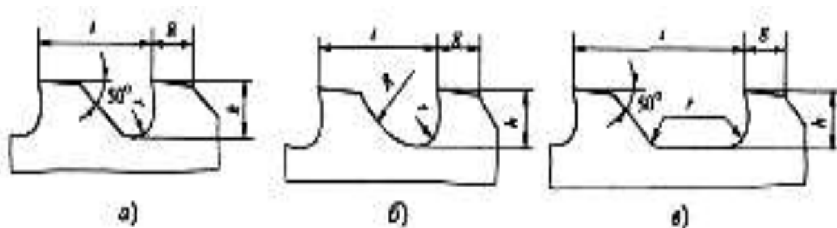
7.4-rasm. Kesuvchi tishlar va qirindi kanavkalarining profili: a – to'g'ri chiziqli; b – egri chiziqli; v – uzaytirilgan shaklli kanavkali
