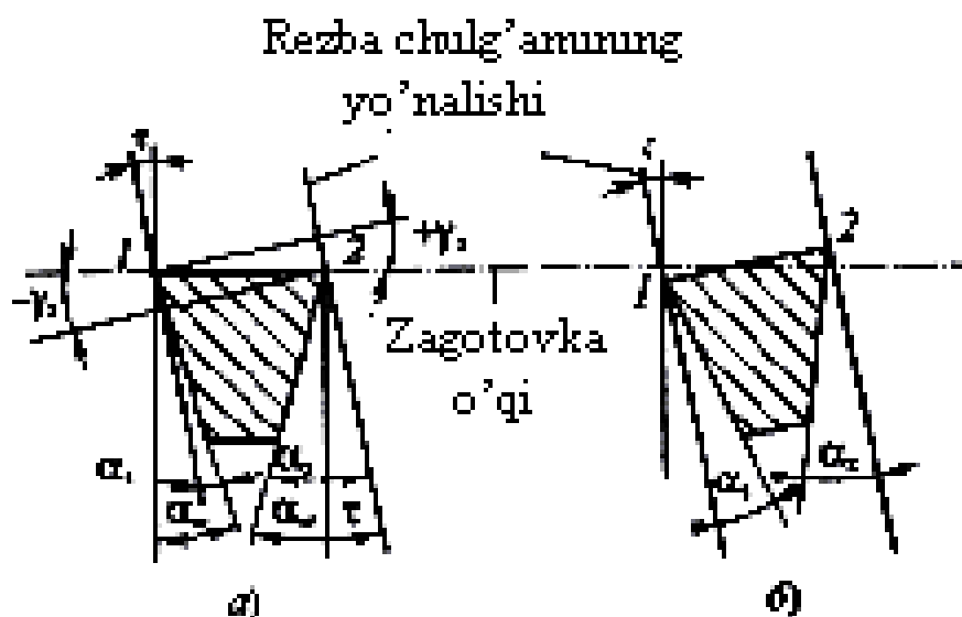
8.2-rasm. Katta ko'tarish burchagi \tau ga ega bo'lgan rez'balarni kesishda strejenli kesikchlarni o'rnatish sxemalari: a – oldingi qirra zagotovkasining o'q bo'ylama yuzasida joylashgan; b – oldingi burchak rez'ba cho'lg'amlariga perpendikulyar joylashgan
