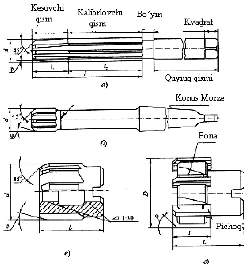
5.1-rasm. Tsilindrsimon razvyortkalar: a – dastaki (qo‘l kuchli); b – mashinali; v – o‘matiluvchi; g – yig‘ma
