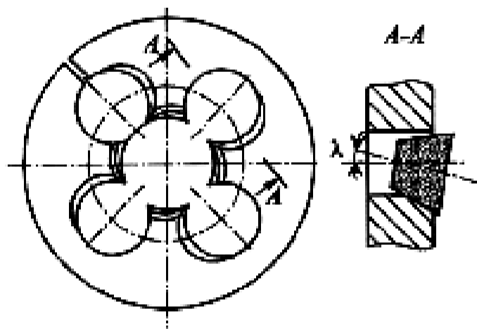
8.24-rasm. Kesuvchi qismni oldingi yuzasi bo'ylab charxlash bilan plashka konstruksiyasini yaxshilash usuli
