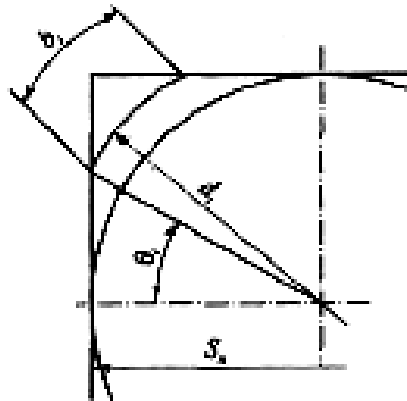
7.8-rasm. Qirrali sidirgichlar kesuvchi qirrasining uzunligini aniqlash sxemasi
