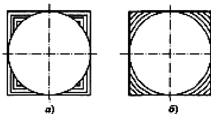
7.6-rasm. Kvadrat shaklli teshiklarga sidirgich bilan ishlov berish sxemalari: a – profili; b – generatorli
