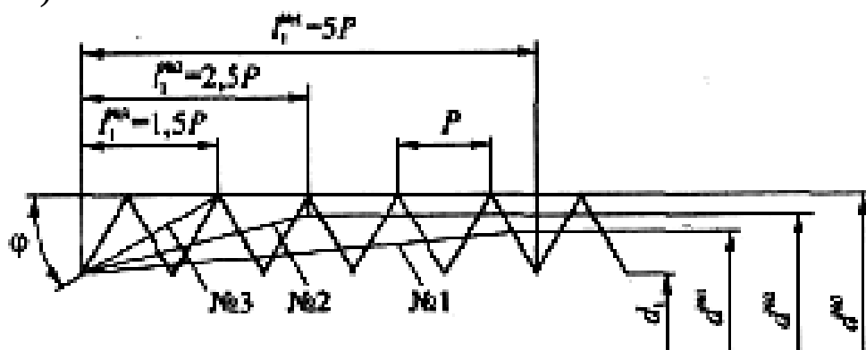
8.13-rasm. Komplektdagi uchta metchiklar orasidagi qo'yimni taqsimlanishi
