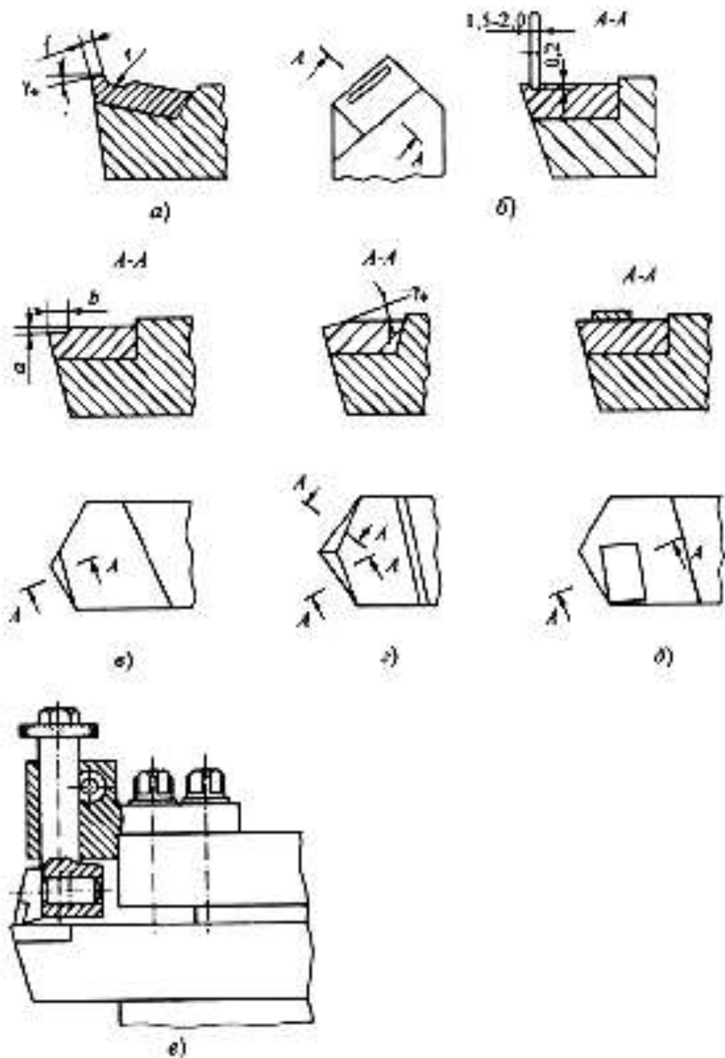
2.7-rasm. Qirindini sindirish usullari: a, b – cho‘kmalar (lunka); v – faska; g – faska ( \gamma_f < 0 ); d – o‘rnatiluvchi sozlanmaydigan plastina; ye – sozlanuvchi qirindi sindirgich
