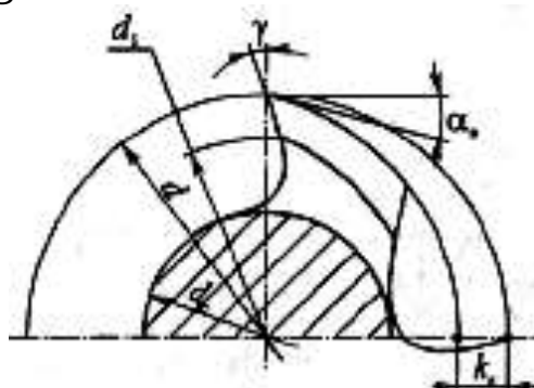
8.14-rasm. Metchik kesuvchi qismi tishlarining geometrik parametrlari
