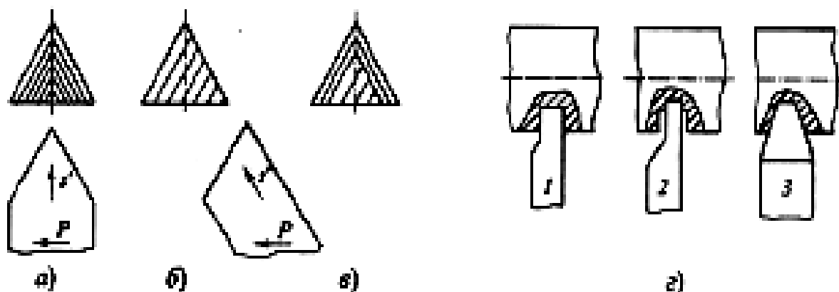
8.3-rasm. Rez'balarni kesishda qo'llaniladigan kesish sxemalari: a – profilli; b – generatorli; v – kombinatsiyalashgan; g – trapetsiyasimon rez'balarni kesish uchun
