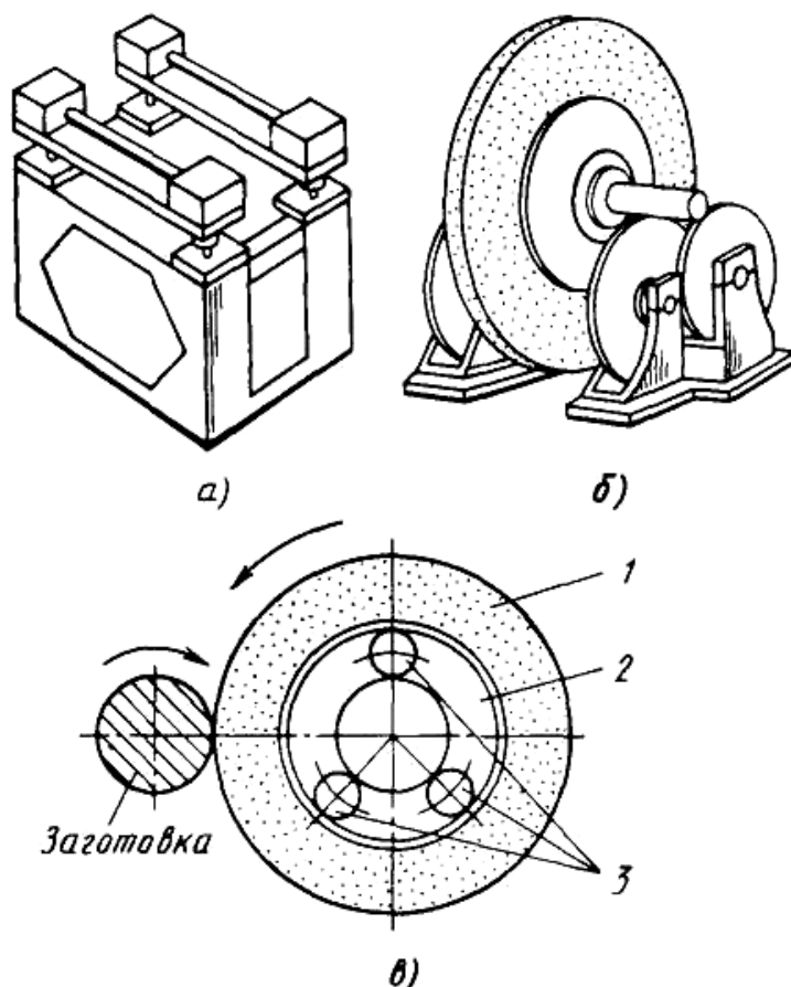
25.5-rasm. Muvozanatlash uchun qurilmalar (a,b) va avtomatik ravishda muvozanlovchi moslamaning sxemasi (v)
