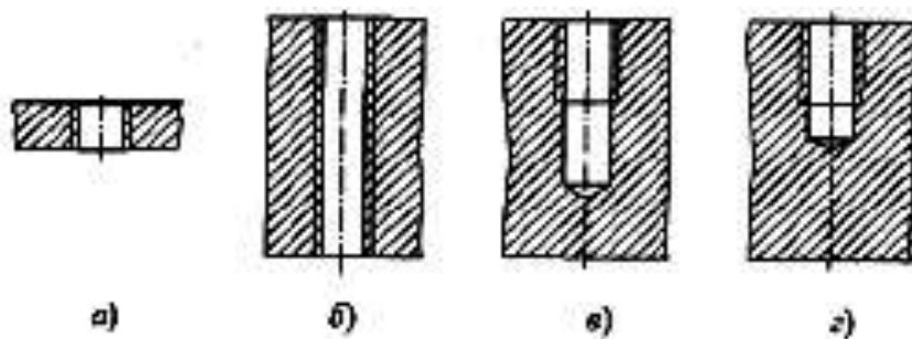
8.12-rasm. Metchiklar yordamida rez'ba kesish uchun teshik turlari: a – kalta ochiq; b – uzun ochiq; v – metchik ko'p masofaga chiquvchi berk; g – kalta berk
