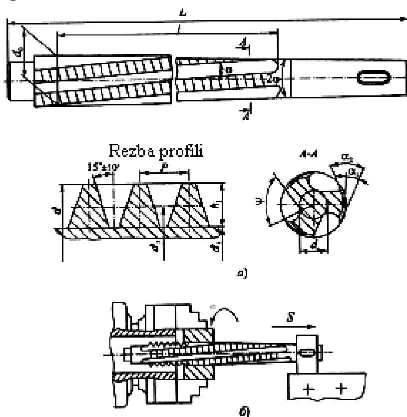
8.19-rasm. Metchik-sidirgich: a – konstruktsiyasi; b – ichki rez'bani sidirish sxemasi
