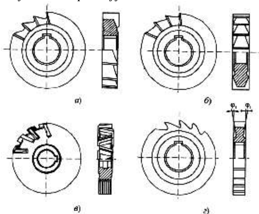
6.3-rasm. Diskli frezalarning turlari:
