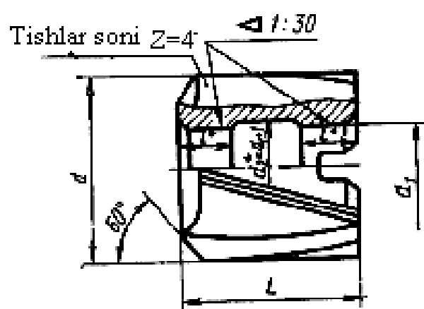
4.2-rasm. Tsilindrsimon zenkerlar: a, b – quyuqli; v – oʻrnatiluvchi
