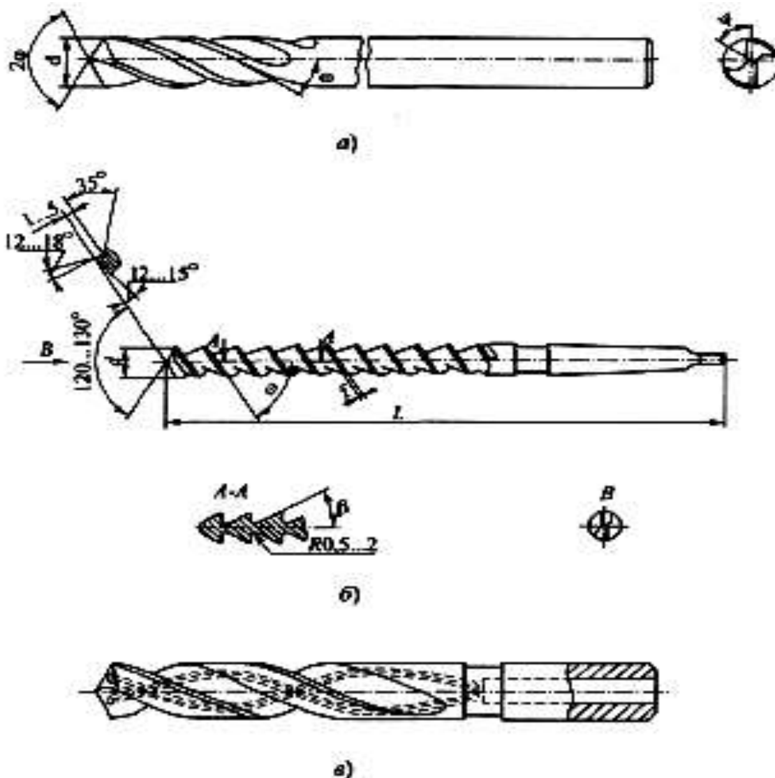
3.9-rasm. Chuqur teshiklar uchun spiral parmalar: a - quyruq qismi uzaytirilgan to'rt lentali; b – ichki sovitish teshikli
