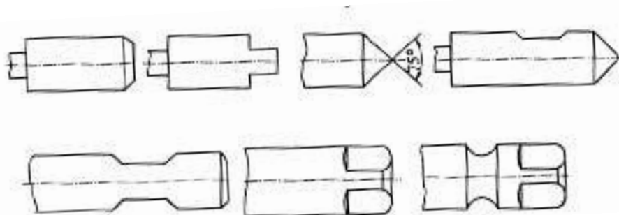
1.4-rasm. Kesuvchi asboblarni tsilindrsimon quyruq qismlarining turi
