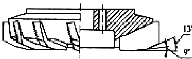
6.5-rasm. Toretsli – konussimon yig'ma freza
