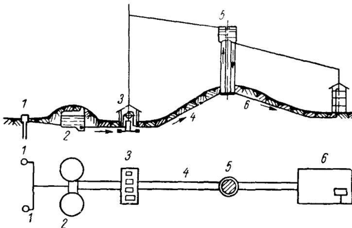
Расм.1.2.Ер ости манбасидан сув таъминоти тизимининг тасвири
