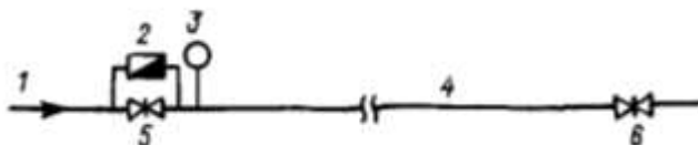
Расм 4.5. Манометр ёрдамида сув йуқолишини аниқлаш тасвири
